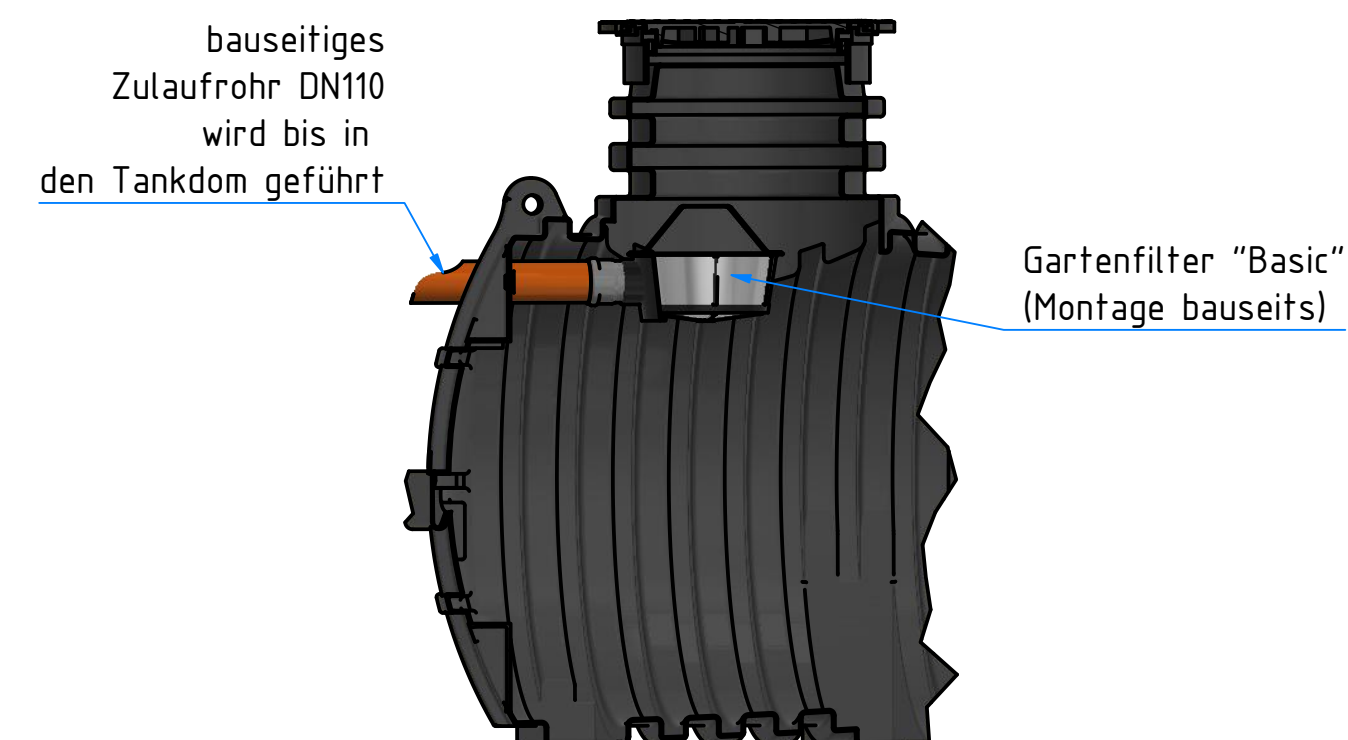
A-A ( 1 : 20 ) Schnitt durch den Dombereich
