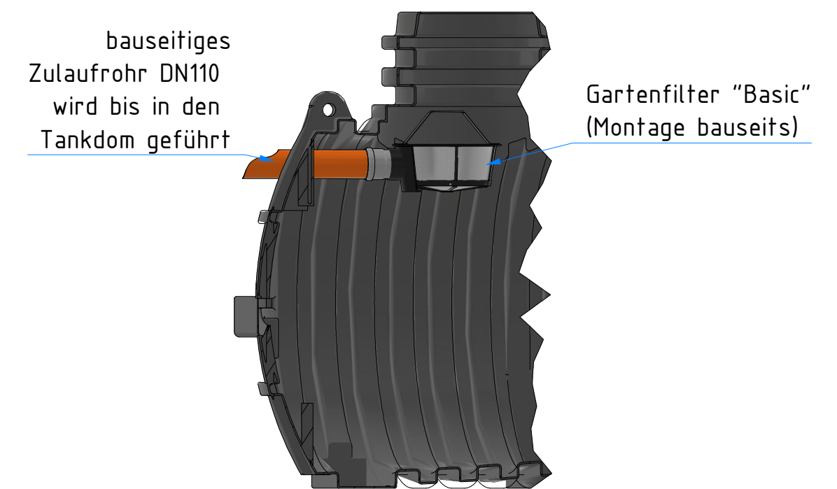
B-B ( 1 : 20 ) Schnitt durch den Dombereich
