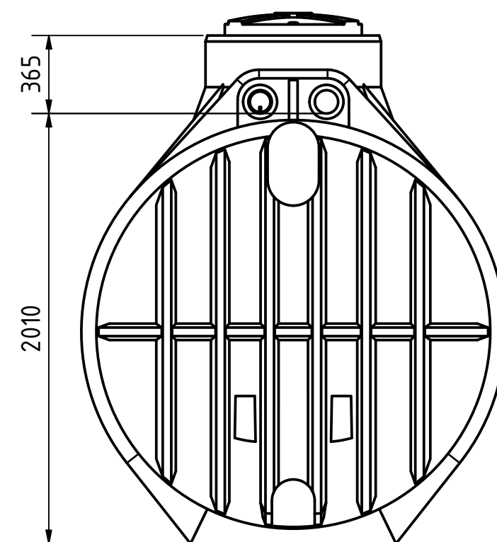
B-B ( 1 : 25 ) Schnitt durch den Dombereich
