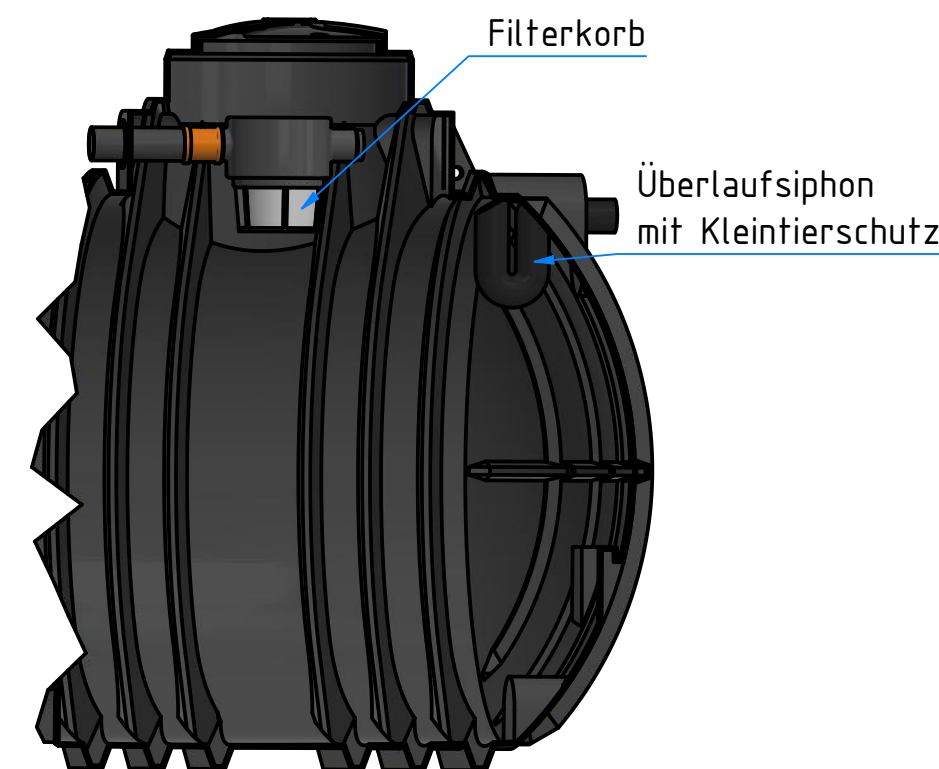
B-B ( 1 : 25 ) Schnitt durch den Dombereich
