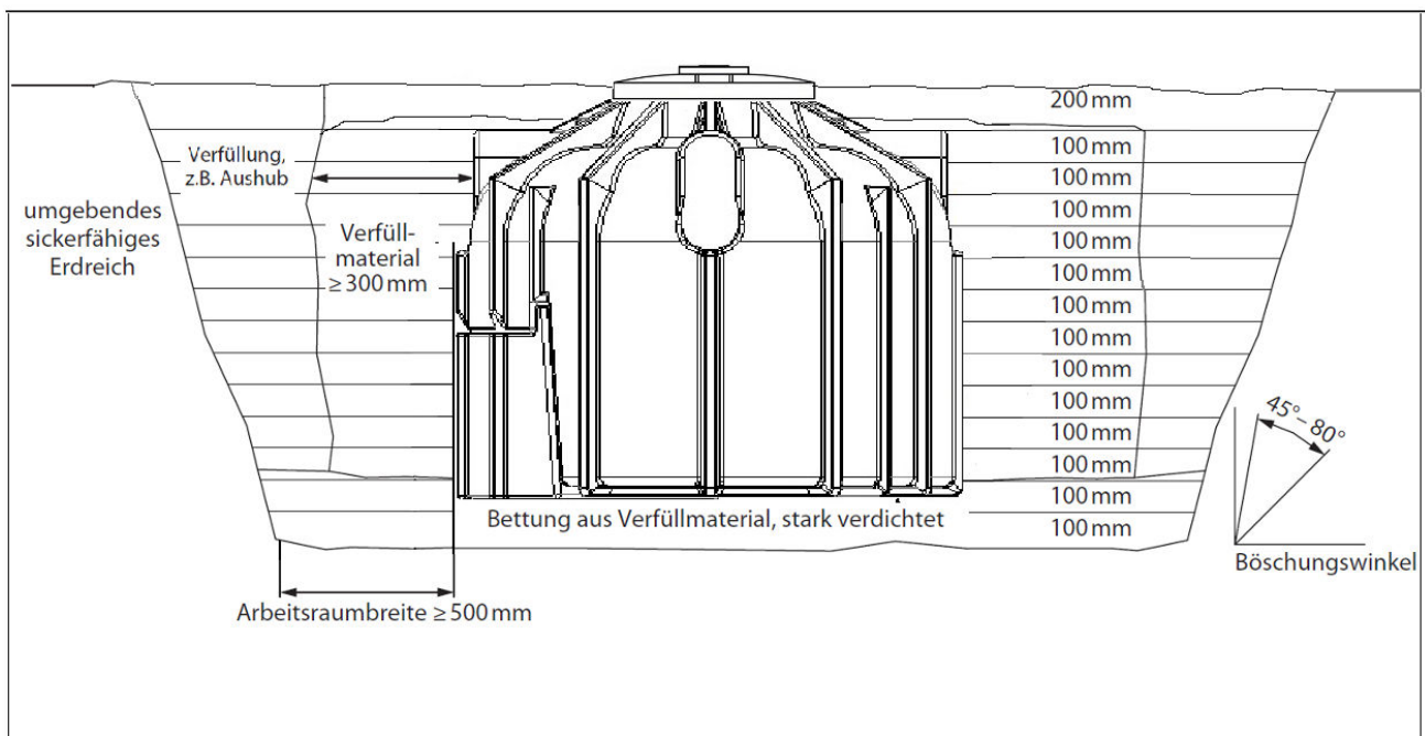
Abbildung 4: Ausführung des Einbaus am Beispiel eines Smart 6400 L Erdtanks mit Basic Abdeckung
