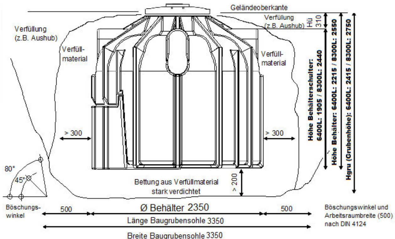
Abbildung 2: Einbaugrößen
