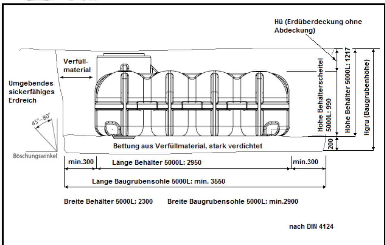
Abbildung 2: Einbaugrößen
