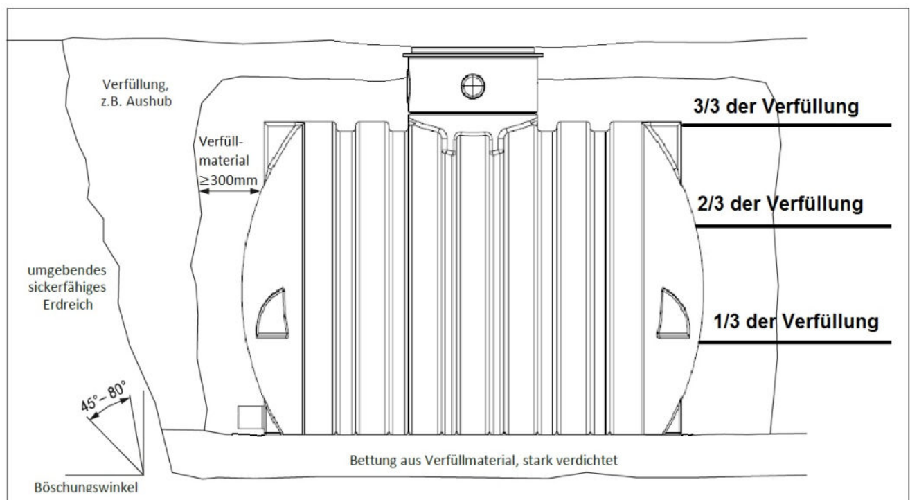
Abbildung 4: Ausführung des Einbaus am Beispiel eines Smart 4000 L Erdtanks mit Tankabdeckung Basic
