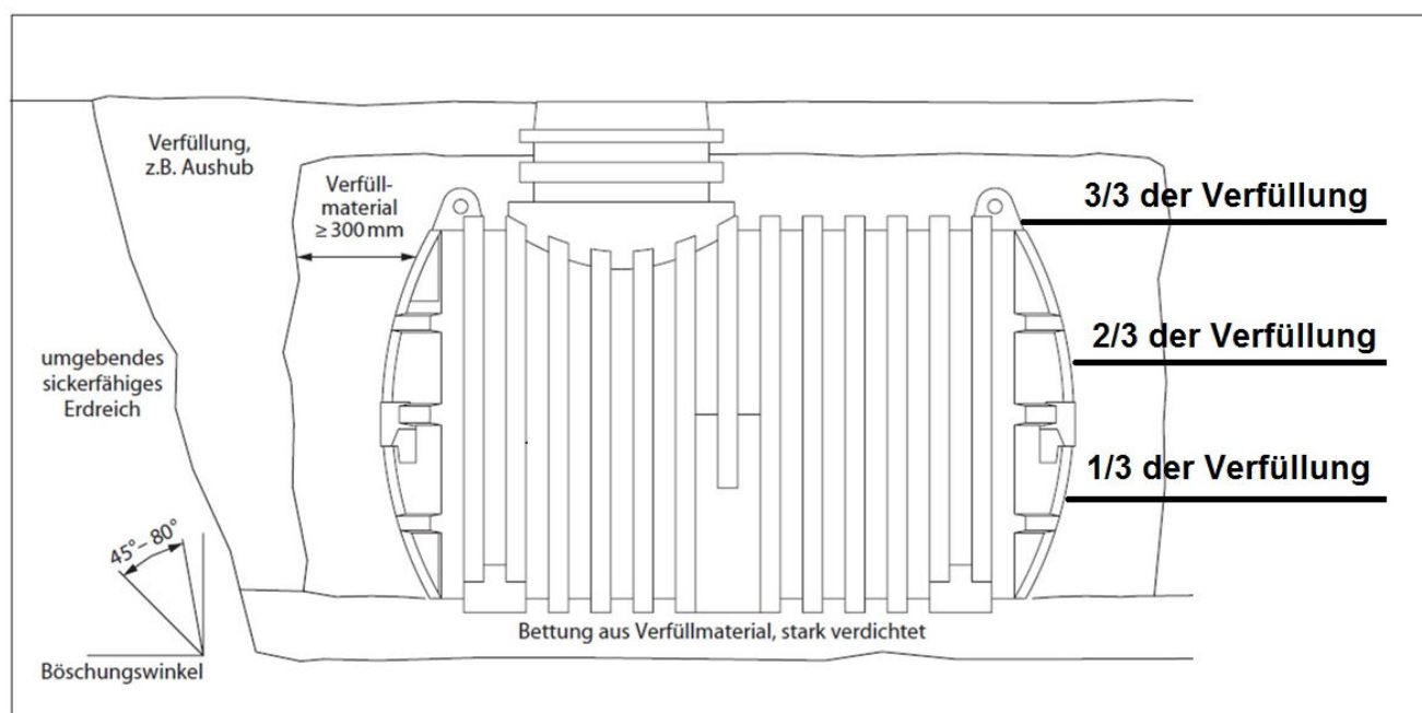
Abbildung 3: Ausführung des Einbaus am Beispiel eines Pluvo 3300 L Erdtanks mit Tankabdeckung Basic
