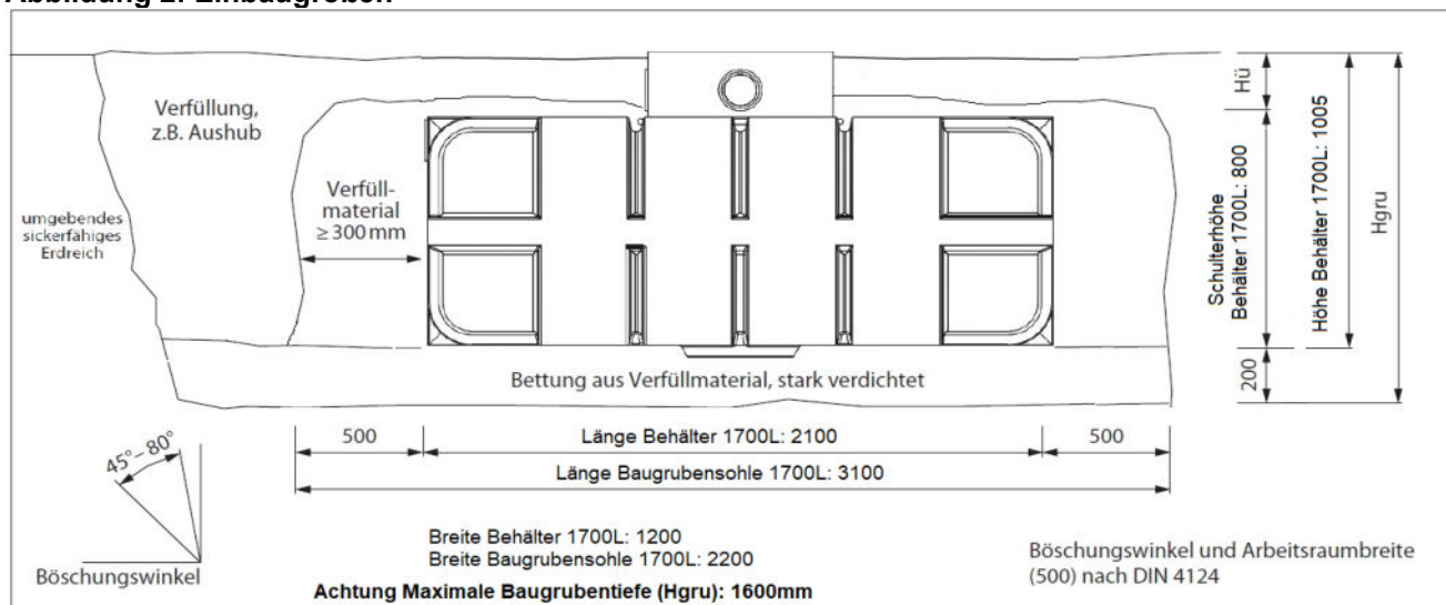
Abbildung 2: Einbaugrößen
