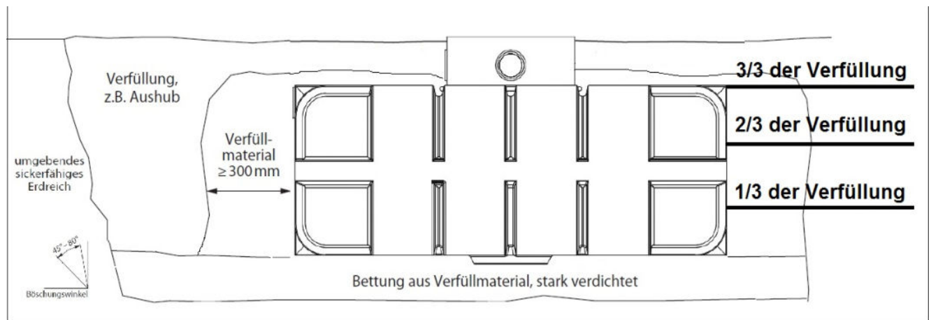
Abbildung 4: Ausführung des Einbaus am Beispiel eines Smart 1700 L Flachtanks mit Tankabdeckung Basic
