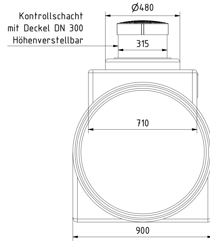
Frontansicht
