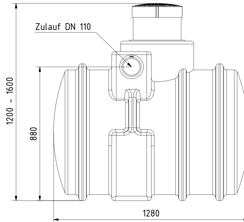
Seitenansicht
