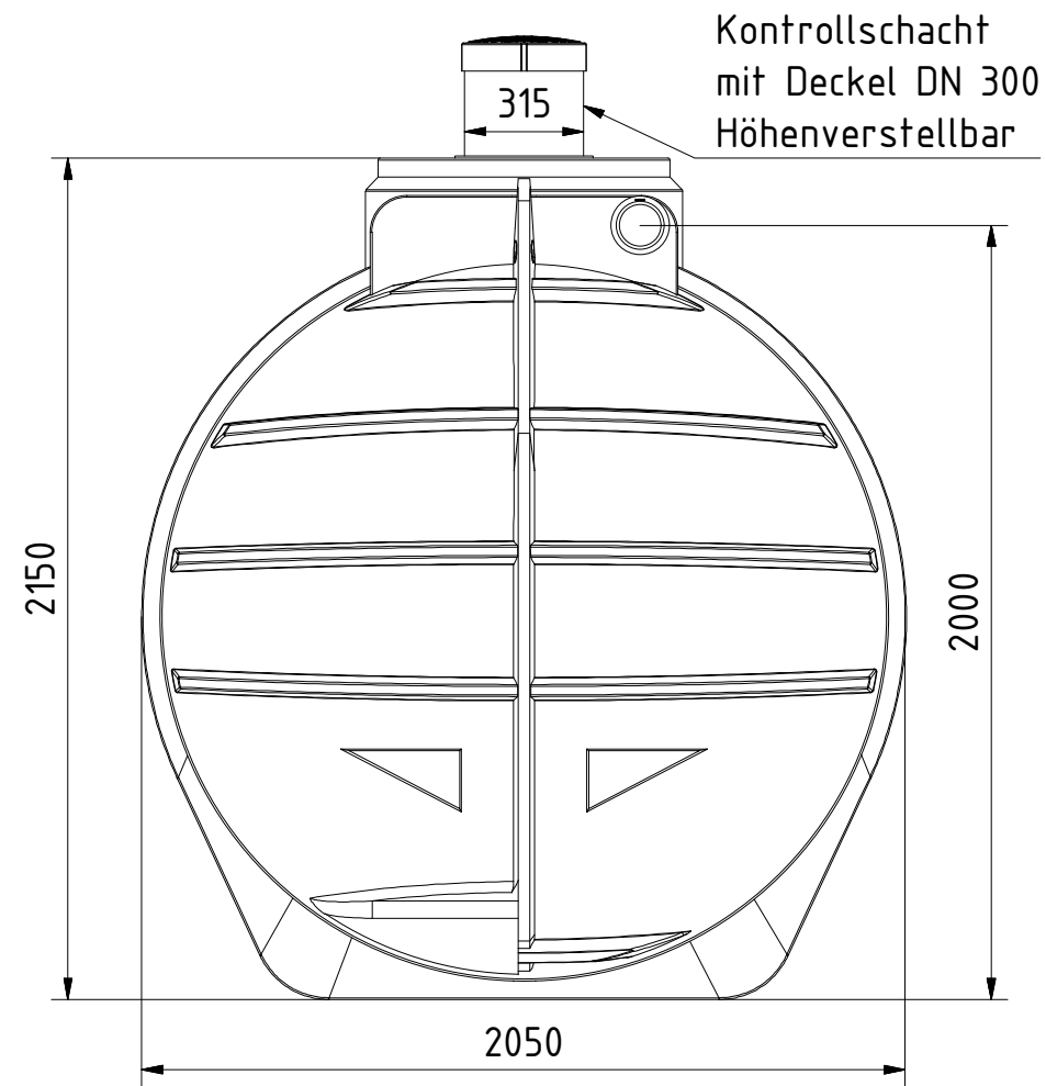
Frontansicht
