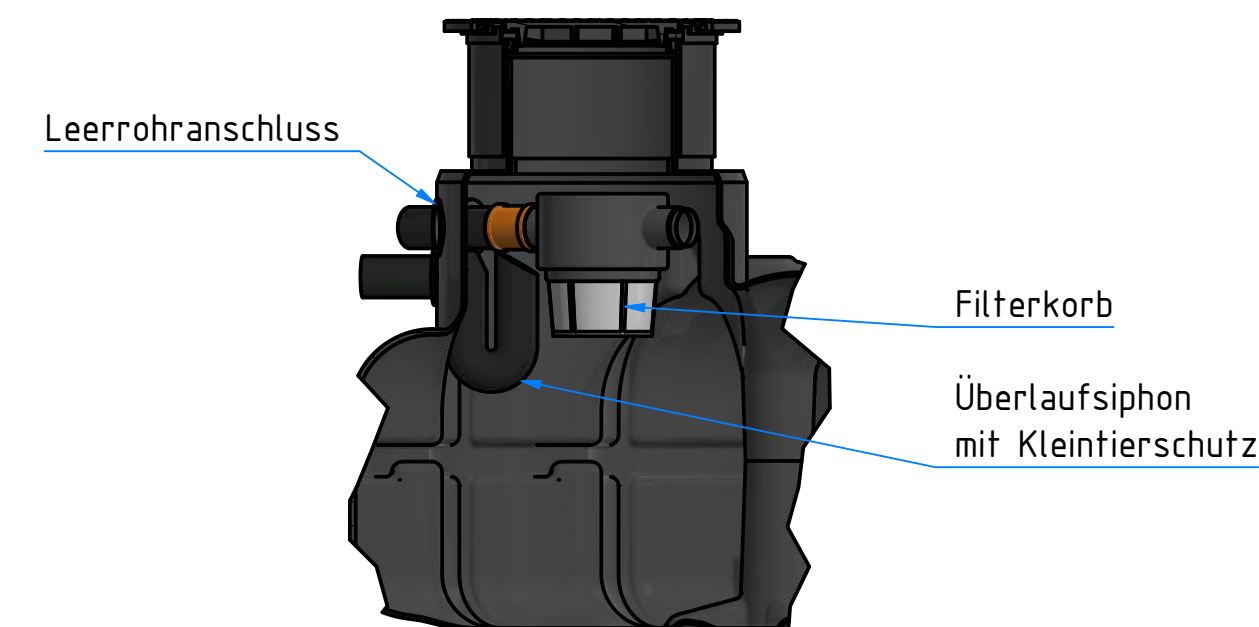
A-A ( 1 : 20 ) Schnitt durch den Dombereich
