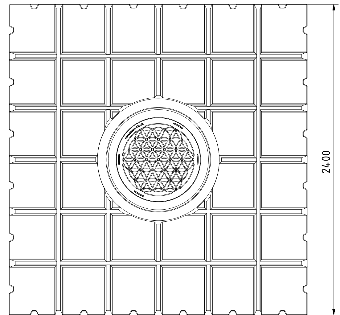
Draufsicht
