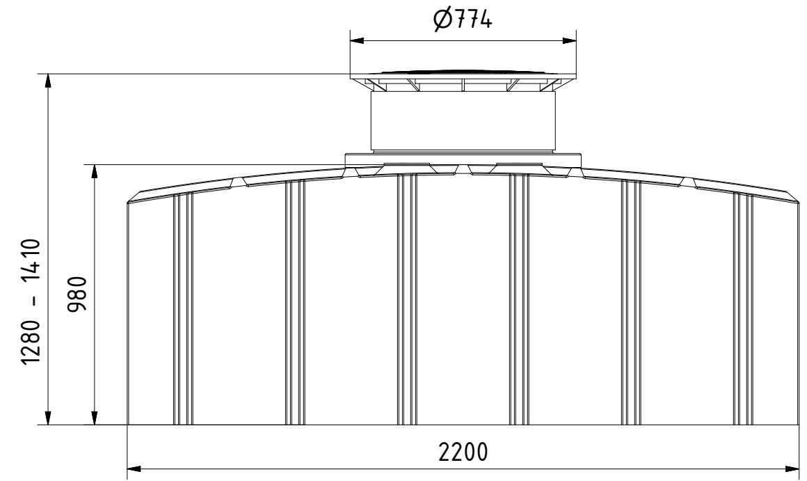
Seitenansicht
