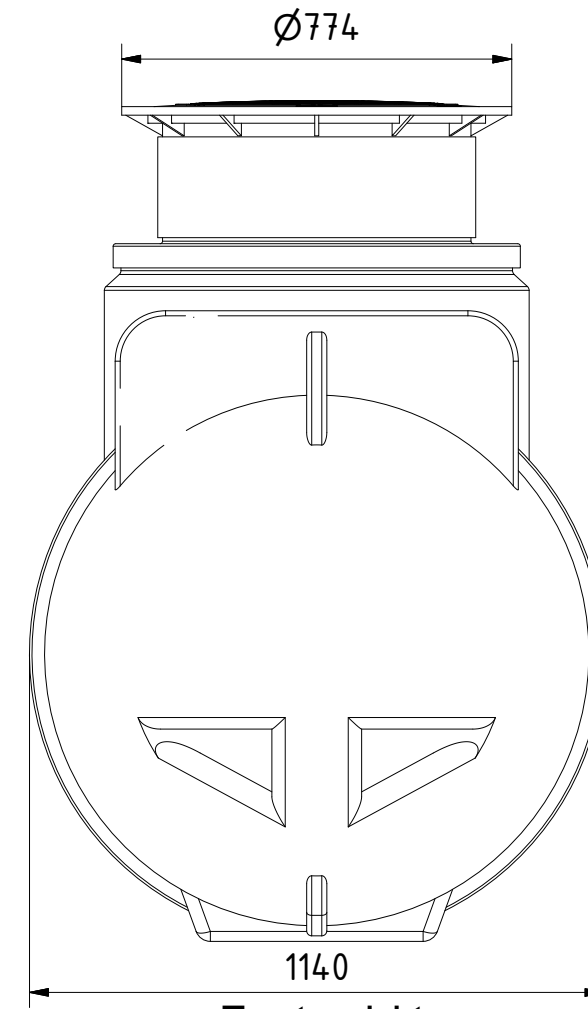
Frontansicht
