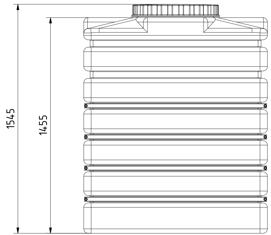
Seitenansicht
