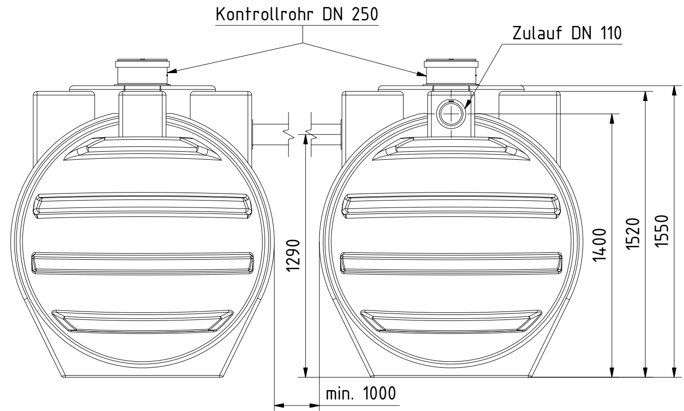
Frontansicht
