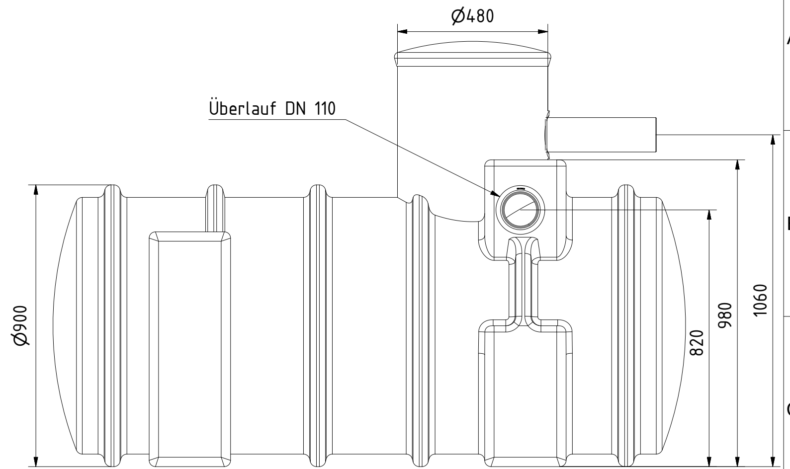
Seitenansicht links
