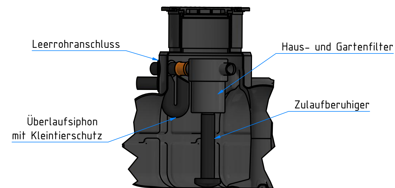
A-A ( 1 : 20 ) Schnitt durch den Dombereich
