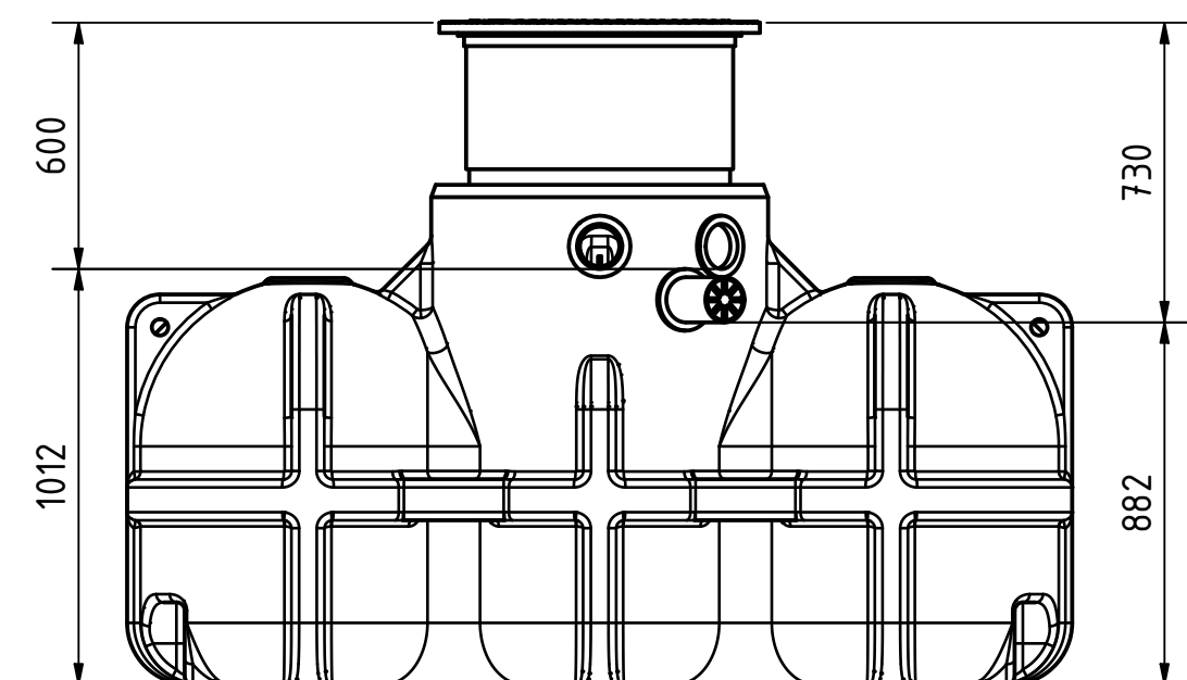
A-A ( 1 : 20 ) Schnitt durch den Dombereich
