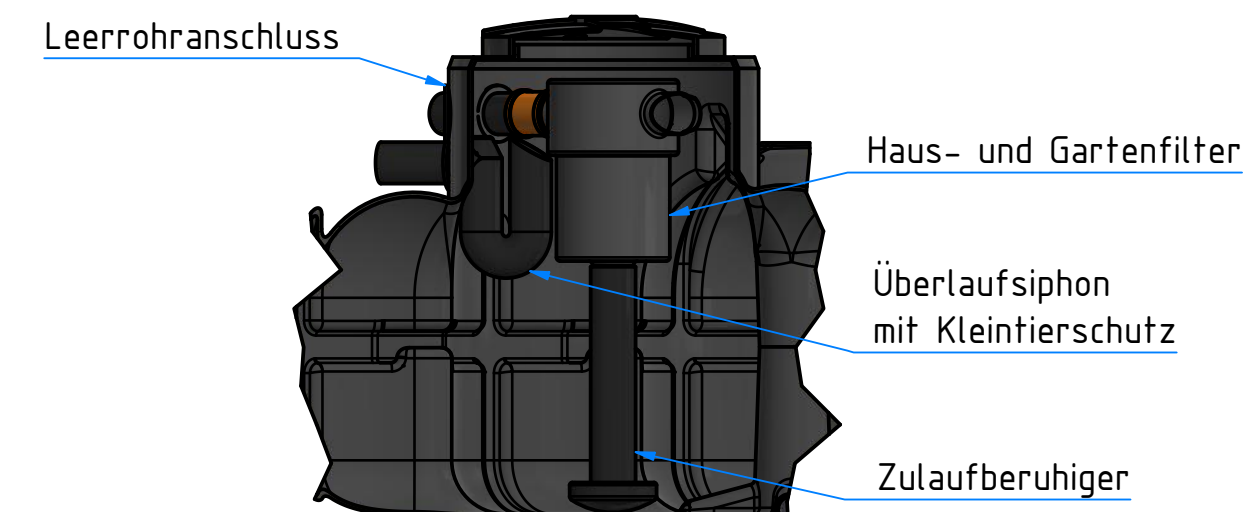
A-A ( 1 : 20 ) Schnitt durch den Dombereich
