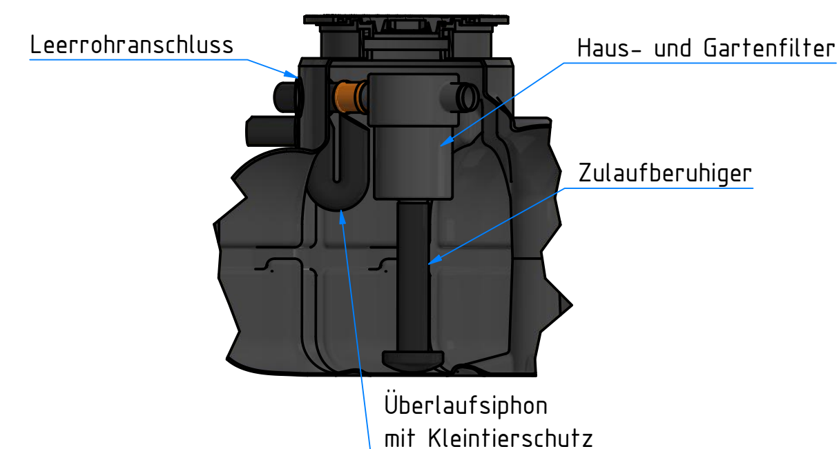
A-A ( 1 : 20 ) Schnitt durch den Dombereich
